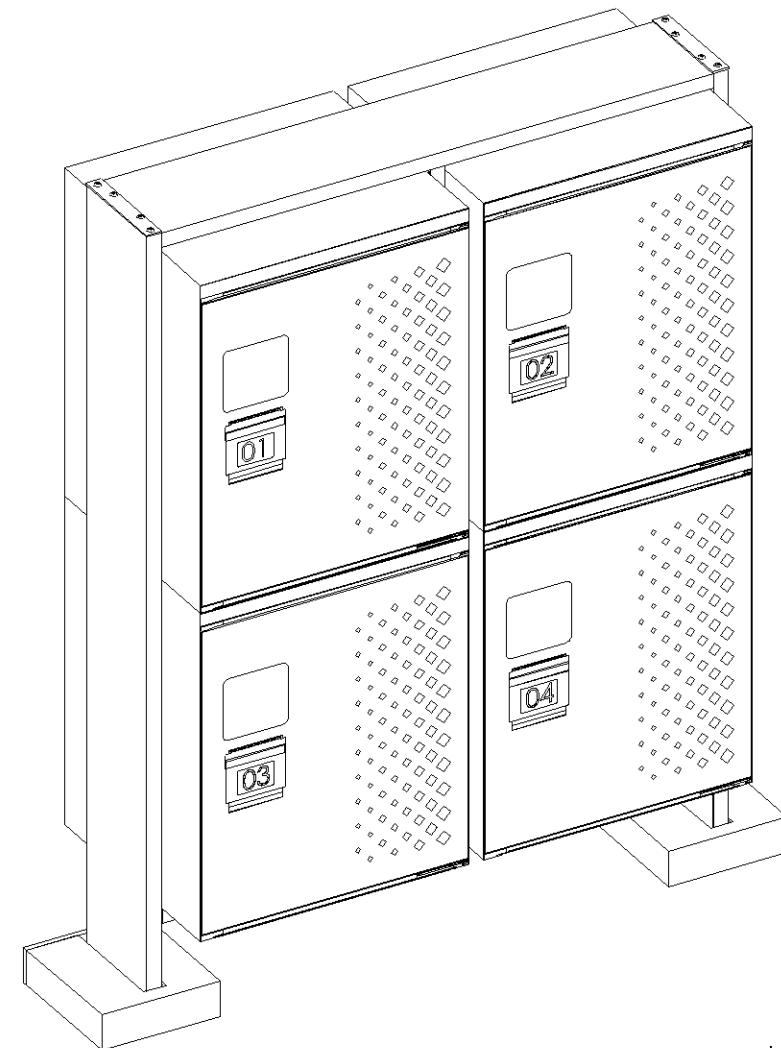
<DTB-S22-S/J> 完成図
